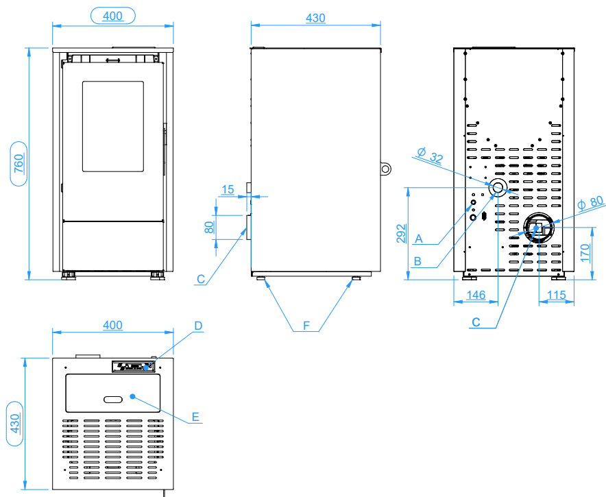
Layout MENSA
